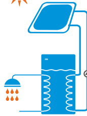
Nyomás alatti napkollektoros rendszer
