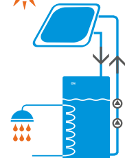
Leeresztő napkollektoros rendszer
